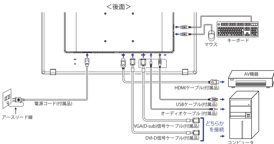
[ 接続例 ]
