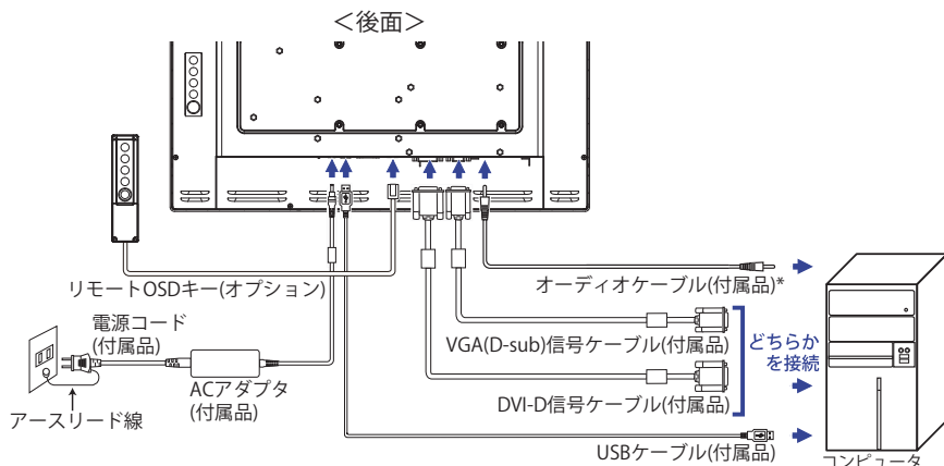
[ 接続例 ]
