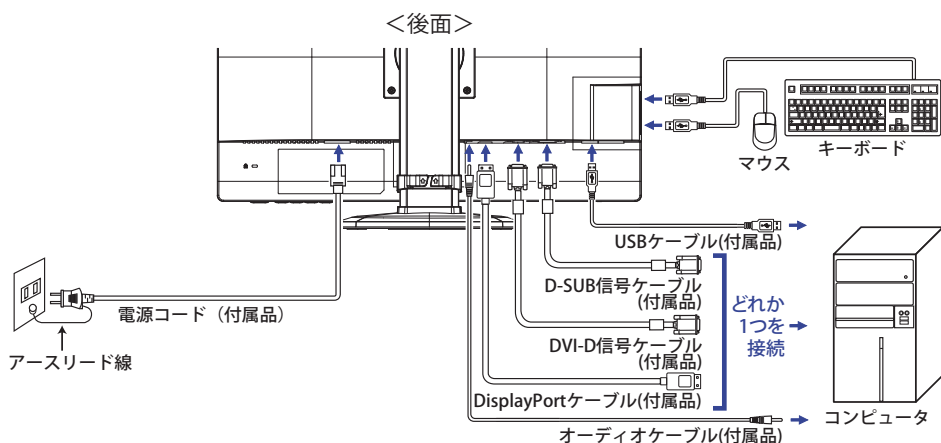
[ 接続例 ]
