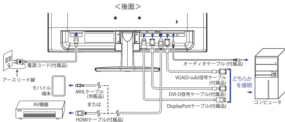
[ 接続例 ]
