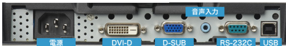
【T1731SR/SAW-2モデルの端子図】
