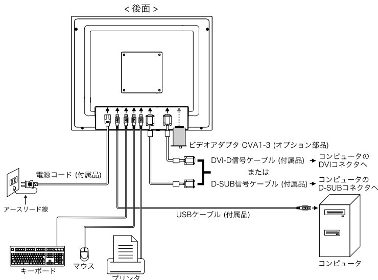
【接続例】
