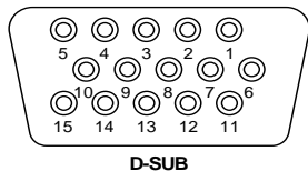
D-SUB
